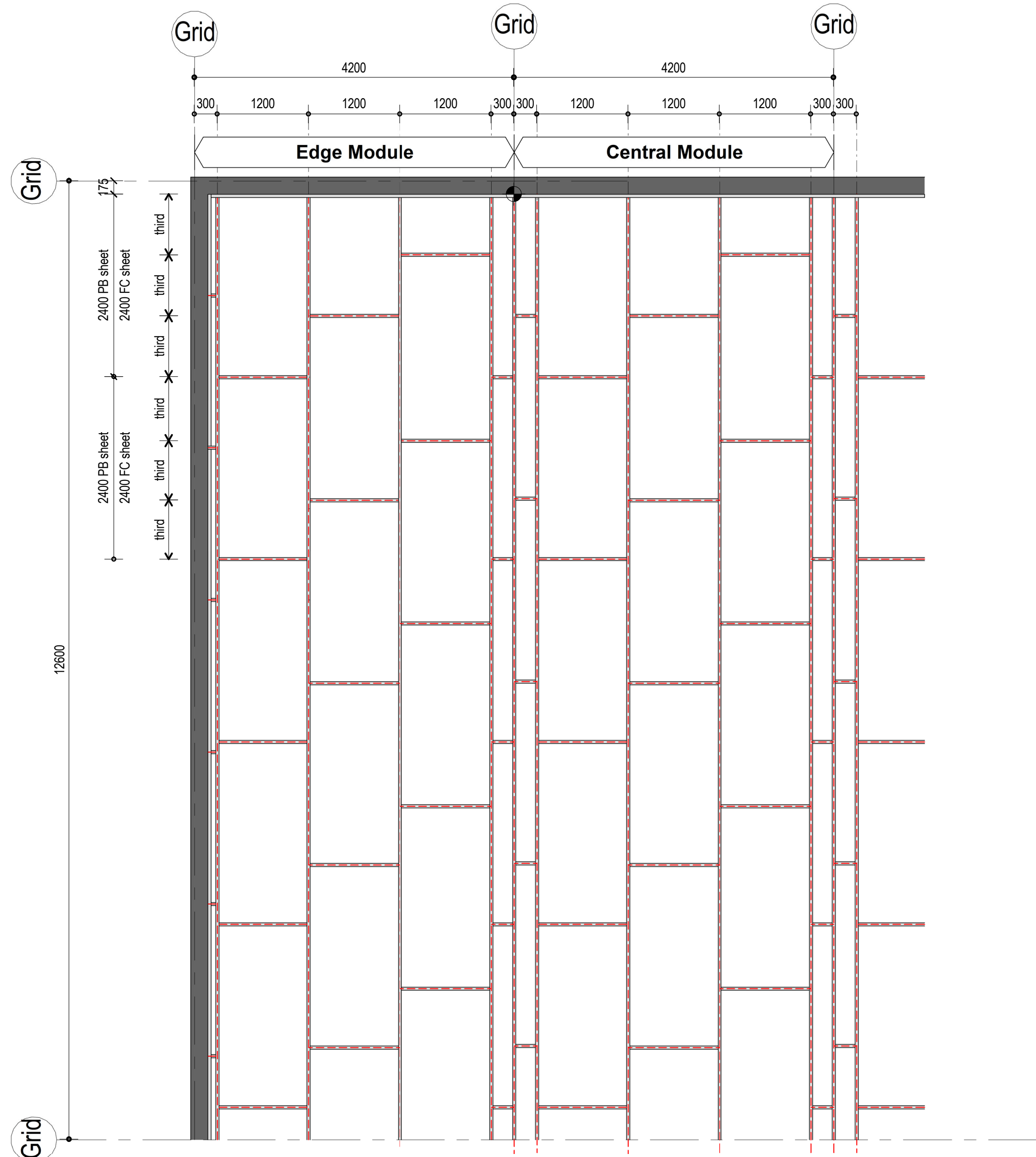
3 Ceiling Batten Setout - Edge 1 : 50
