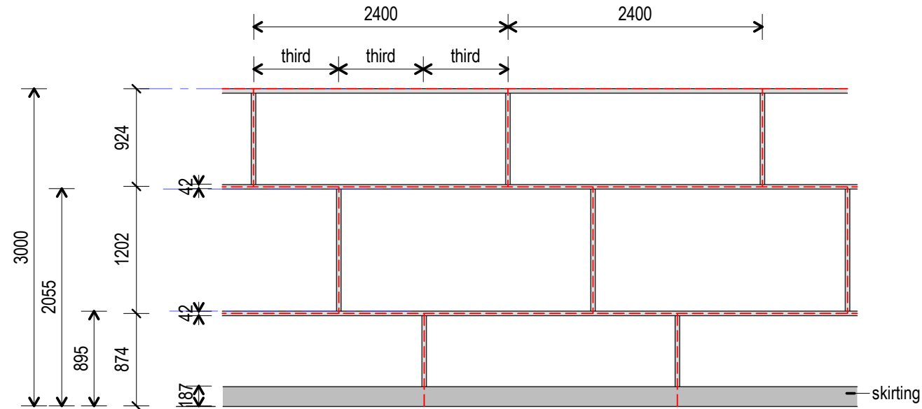
2 Wall Batten Setout - Typ. Horizontal Module 1 : 50
