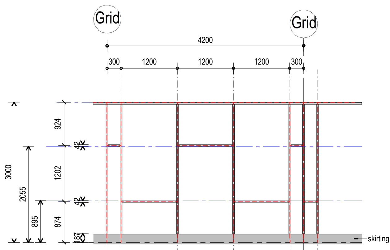
1 Wall Batten Setout - Typ. Vertical Module 1 : 50
